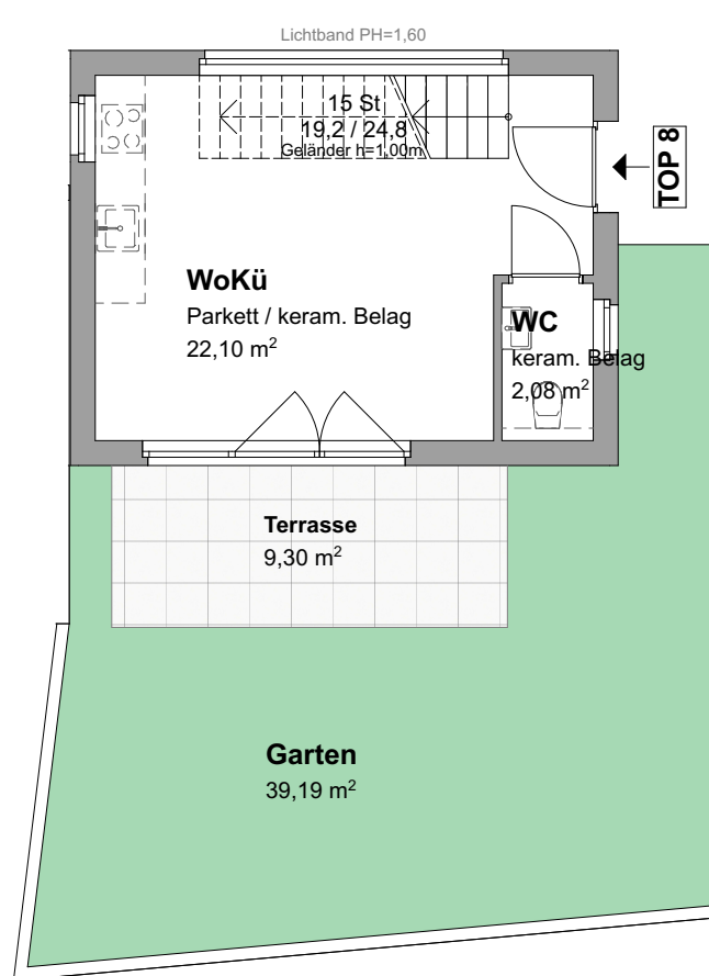
TOP 8 EG M 1:100
